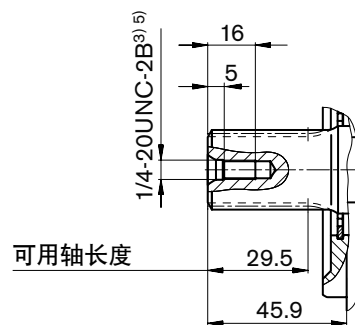
R 花键轴, 1 in 15T 16/32DP 1)2) (SAE J744)
