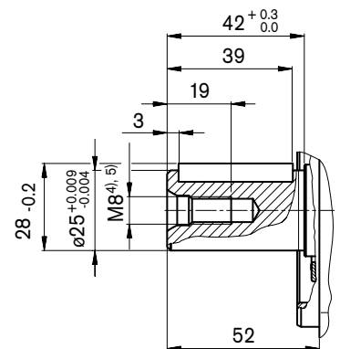
P 平键轴 DIN 6885, A8x7x36
