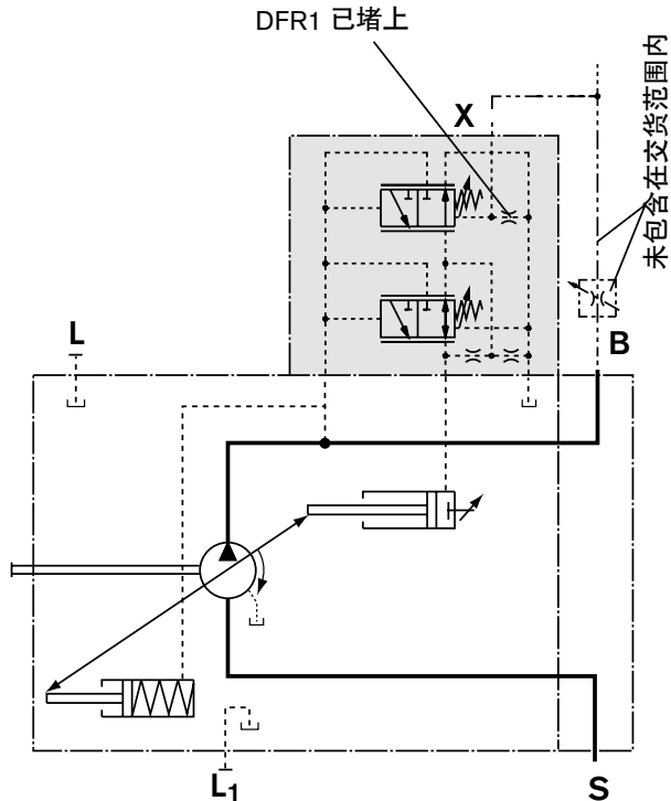
油路图, 规格 140
