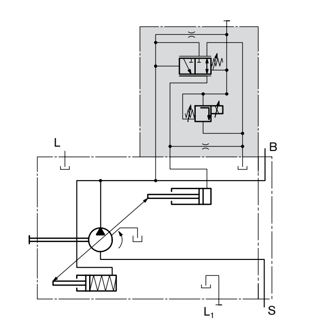
油路图 ER..
