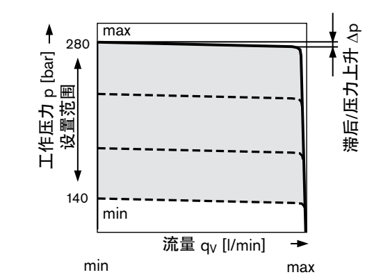
静态流量压力特性 ( n = 1500 rpm; t_{油液} = 50 °C)
