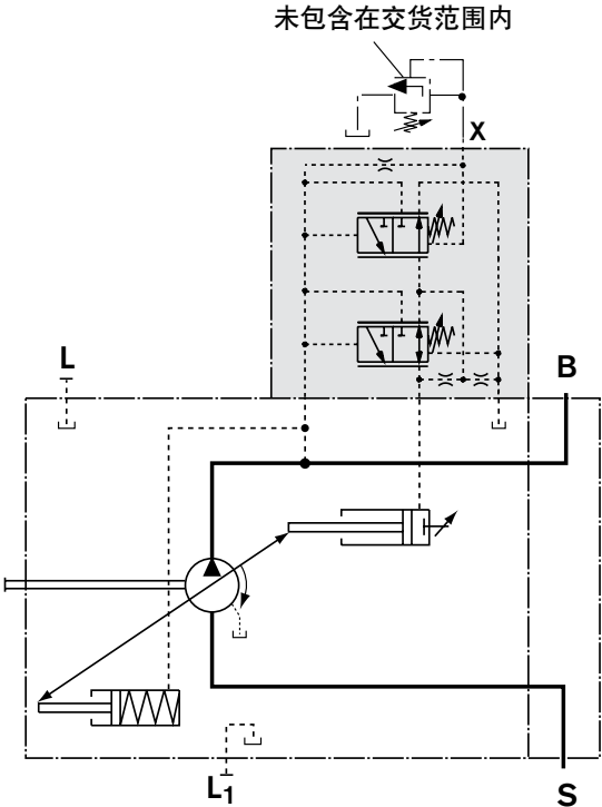
油路图，规格 140
