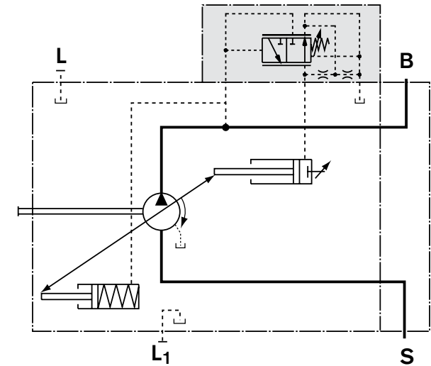
油路图，规格 140
