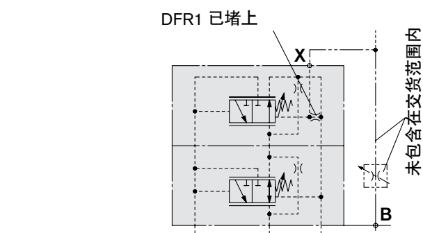
油路图, 规格 140
