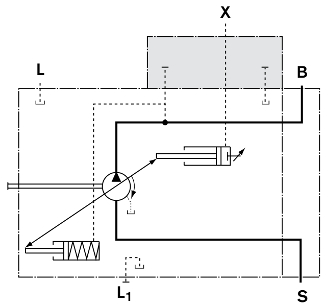
油路图
